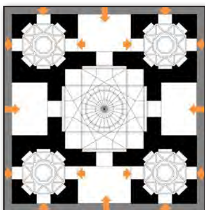
تصویر ۹. بازسازی پلان شربت‌خانه خانقاه سید واقف. نطنز. مأخذ: نگارنده. Fig. 9. Recon- structed Plan of the Sherbet House of Sayed Vaghef Abbey. Natanz. Source: author.
