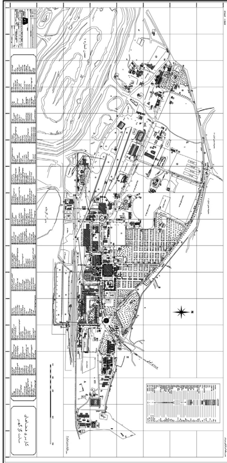
سایت پلان مجتمع معدنی صنعتی گل گهر
